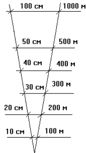
Рис. 9. Угол, образованный одной тысячной
