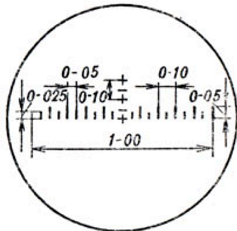
Рис. 12. Сетка бинокля
