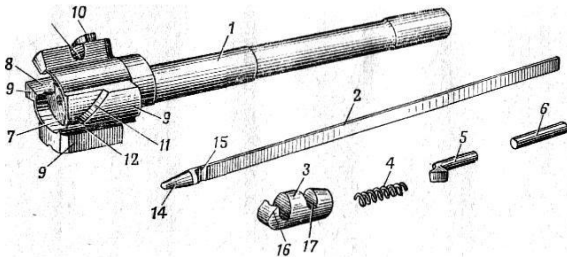
Рис. 20. Затвор:
