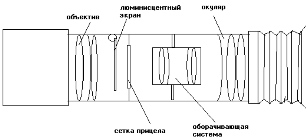
Рис. 29. Оптический прицел ПСО-1: А – механическая часть, Б – оптическая часть
