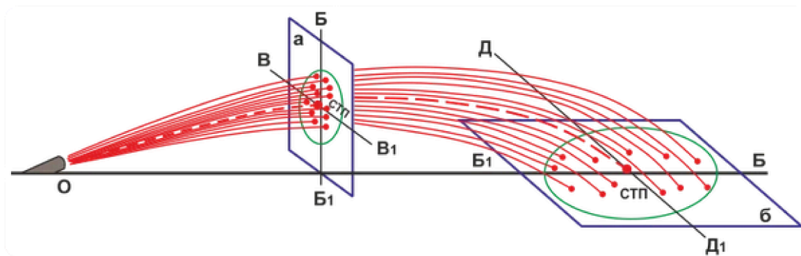
Рис. 7. Сноп траекторий, площадь рассеивания, оси рассеивания: а — в вертикальной плоскости; б — в горизонтальной плоскости; средняя траектория обозначена пунктирной линией; СТП — средняя точка попадания; ВВ1 — ось рассеивания по высоте; ББ1 — ось рассеивания по боковому направлению; ДД1 — ось рассеивания по дальности.
