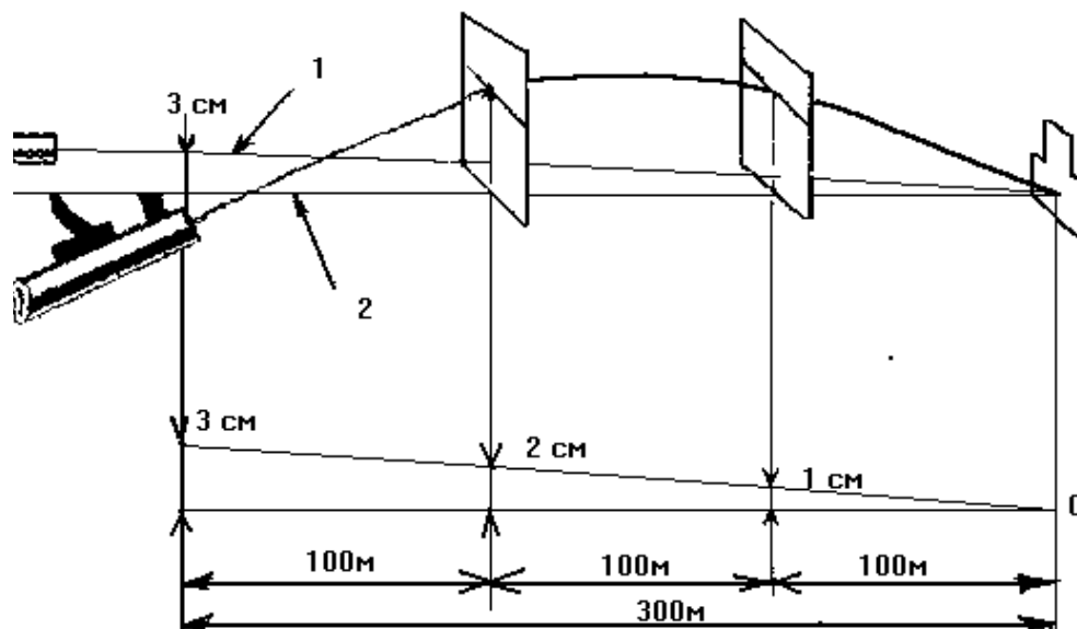
Рис. 35. Схема прицеливания:
