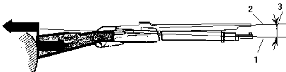
Рис.2. Образование угла вылета при выстреле:
