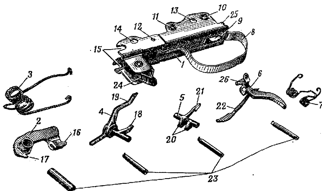
Рис. 21. Ударно-спусковой механизм:
