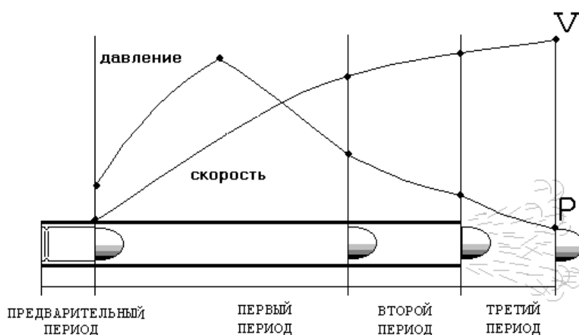
Рис. 1. Изменение давления и скорости пули при ее движении по каналу ствола
