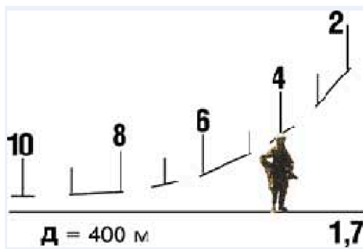
Рис. 10. Определение расстояния до цели по дальномерной шкале прицела ПСО-1
