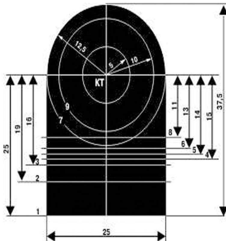
Рис.33. Мишени для приведения СВД к нормальному бою
