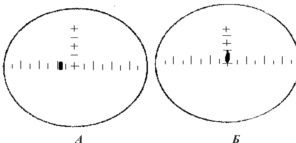
Рис. 13. Определение расстояния с помощью сетки бинокля: А – по ширине цели; Б – по высоте цели.
