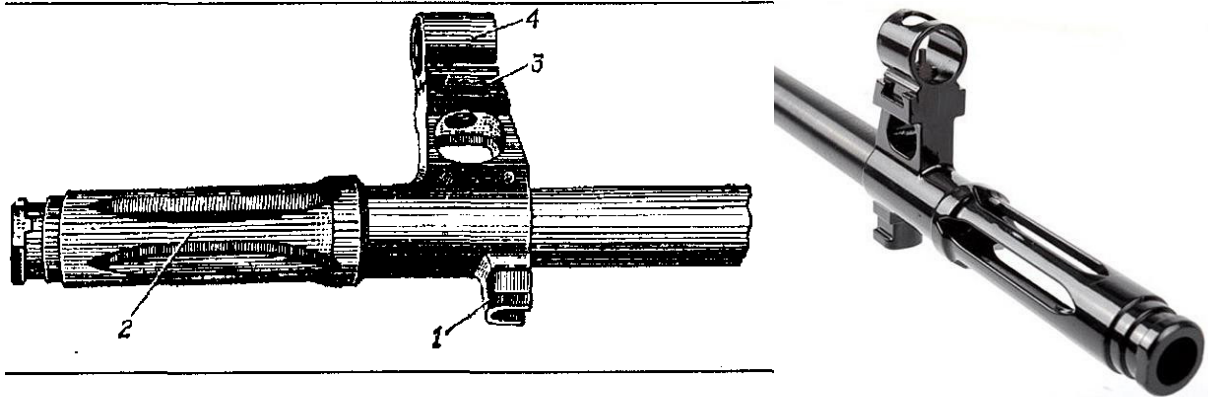
Рис. 17. Основание мушки:
