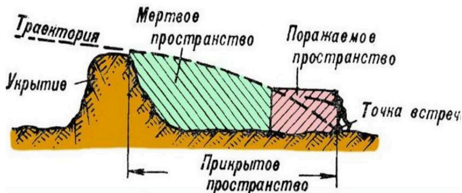
Рис. 6. Мертвое, поражаемое, прикрытое пространство
