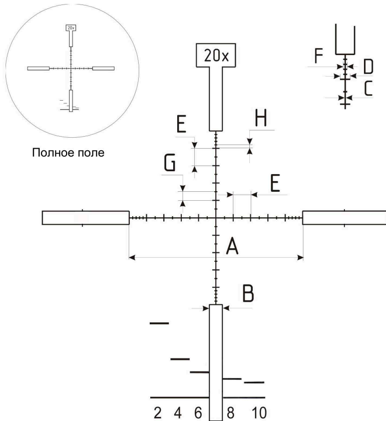
Рис. 37. Сетка прицела DS 5-20x56 MCT
