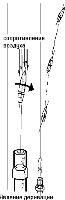
Рис. 4. Явление деривации
