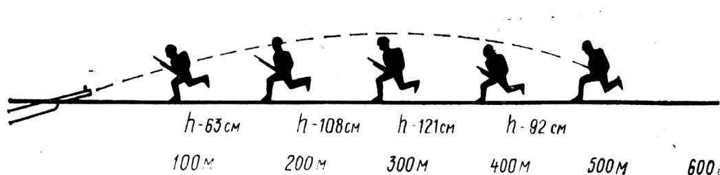
Рис. 5. Прямой выстрел
